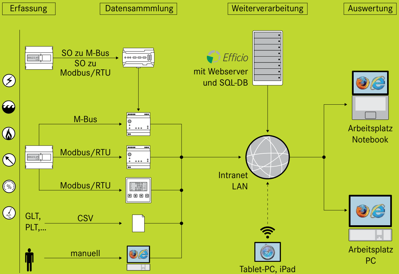
Systemaufbau Efficio
